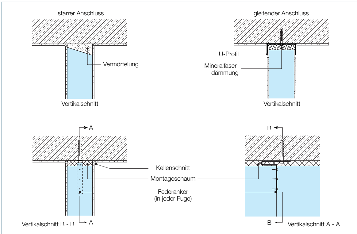
Oberer Anschluss nicht tragender Innenwände aus Porenbetonmauerwerk
